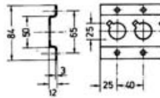
Bėgelis su skylėmis
